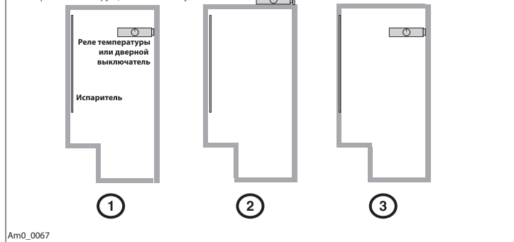
Рис. 4. Варианты конструкции холодильной установки
