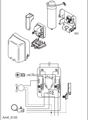
На рисунке 12 показана монтажная схема компрессора с пусковым реле, пусковым конденсатором и устройством защиты электродвигателя, установленным снаружи компрессора.
