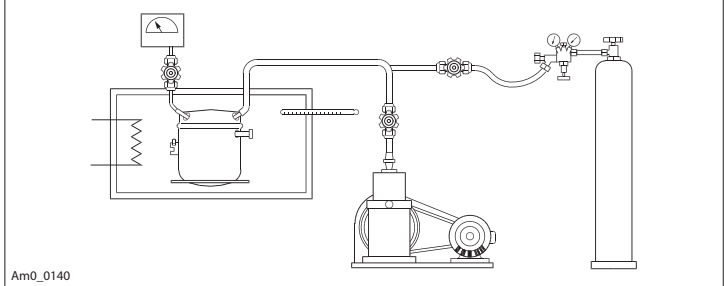
Рис. 20. Осушение компрессора
