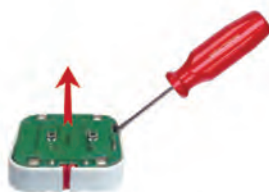
Извлечение платы для замены батарей
