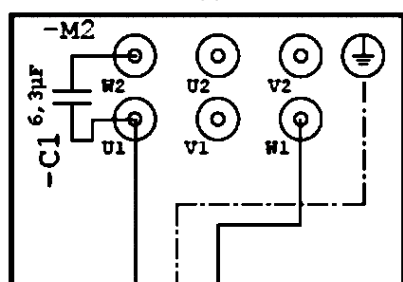
Схема подключения
