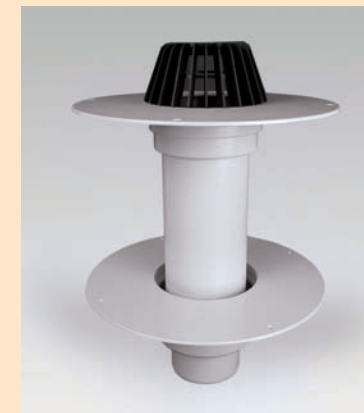
Двухуровневые ПВХ-воронки в сборе S-Gully-Set
