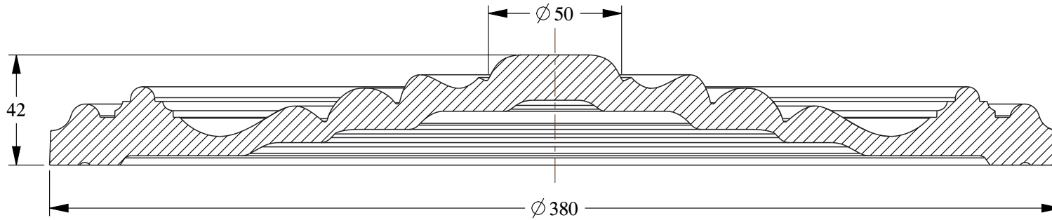
SECTION A-A
