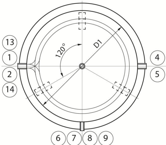
Вид зверху
