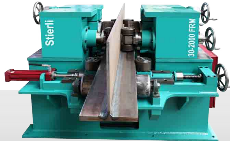
282 Typ 30/2000 FRM
