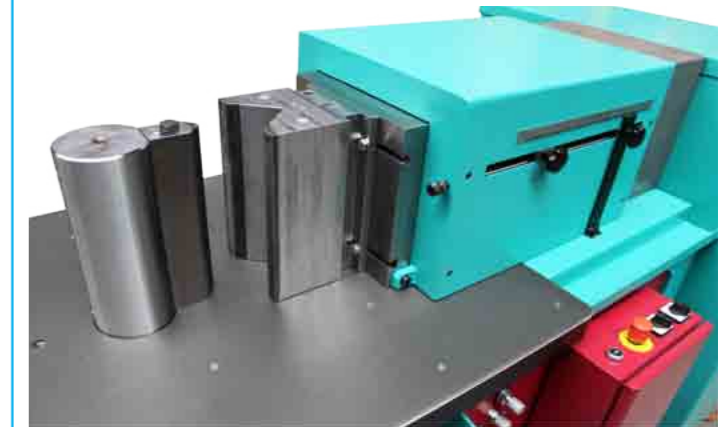
172 Biegestempel und Prisma MW 125 Bending punch and vee-block MW 125
