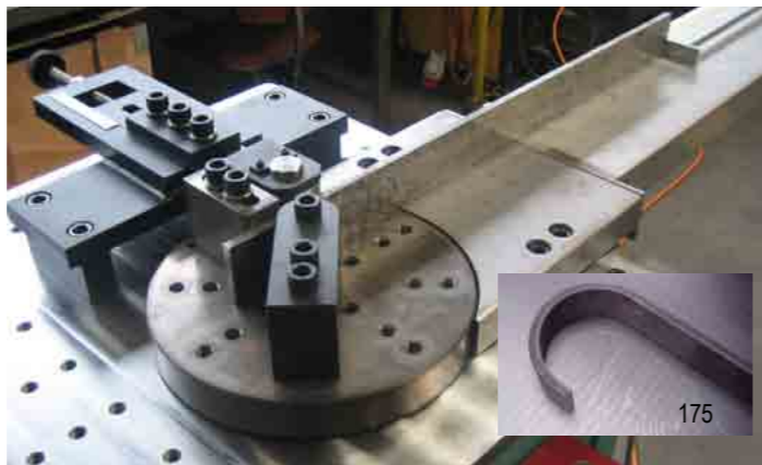
244 Robustes Biegesegment ermöglicht kleine Radien Strong bending pin for smal radius
