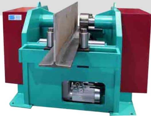
283 Typ 15/2000 + Typ FRM 20/2000FRM
