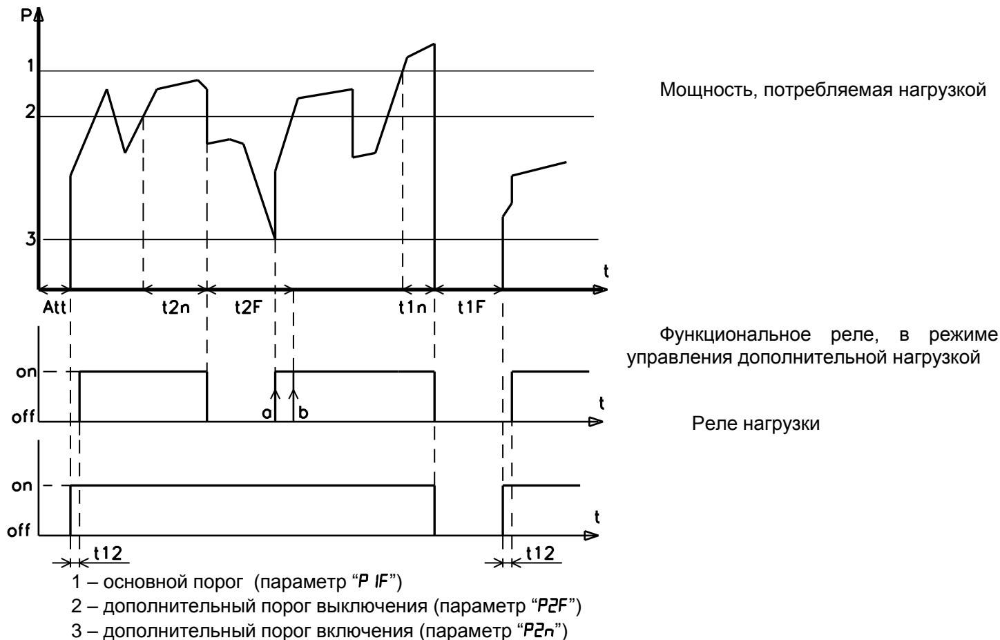
Рисунок 1.3 - Работа OM-310 в режиме ограничения мощности при r_{2r}=2
