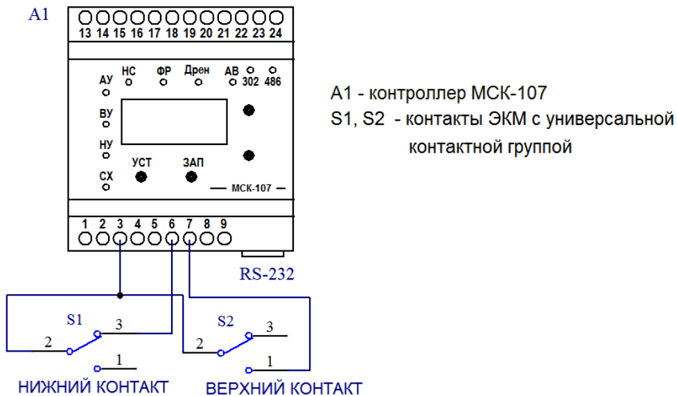
Рисунок 2.2 - Схема подключения датчика давления (ЭКМ)
