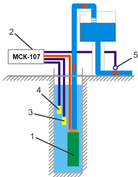
Рисунок 2.4 – Применение MCK-107 в режиме наполнения с датчиком давления
