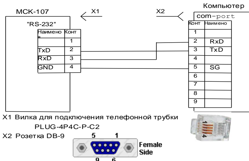
Рисунок 2.7 - Схема подключения МСК-107 к компьютеру
