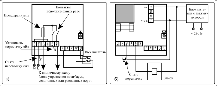
Рисунок 7 Подключение устройства: а) к блокам управления воротами; б) к замкам
