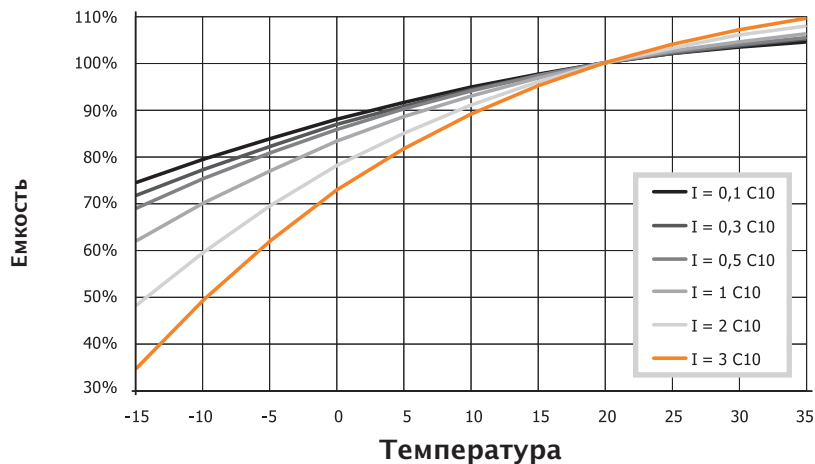
Емкостно-температурная зависимость
