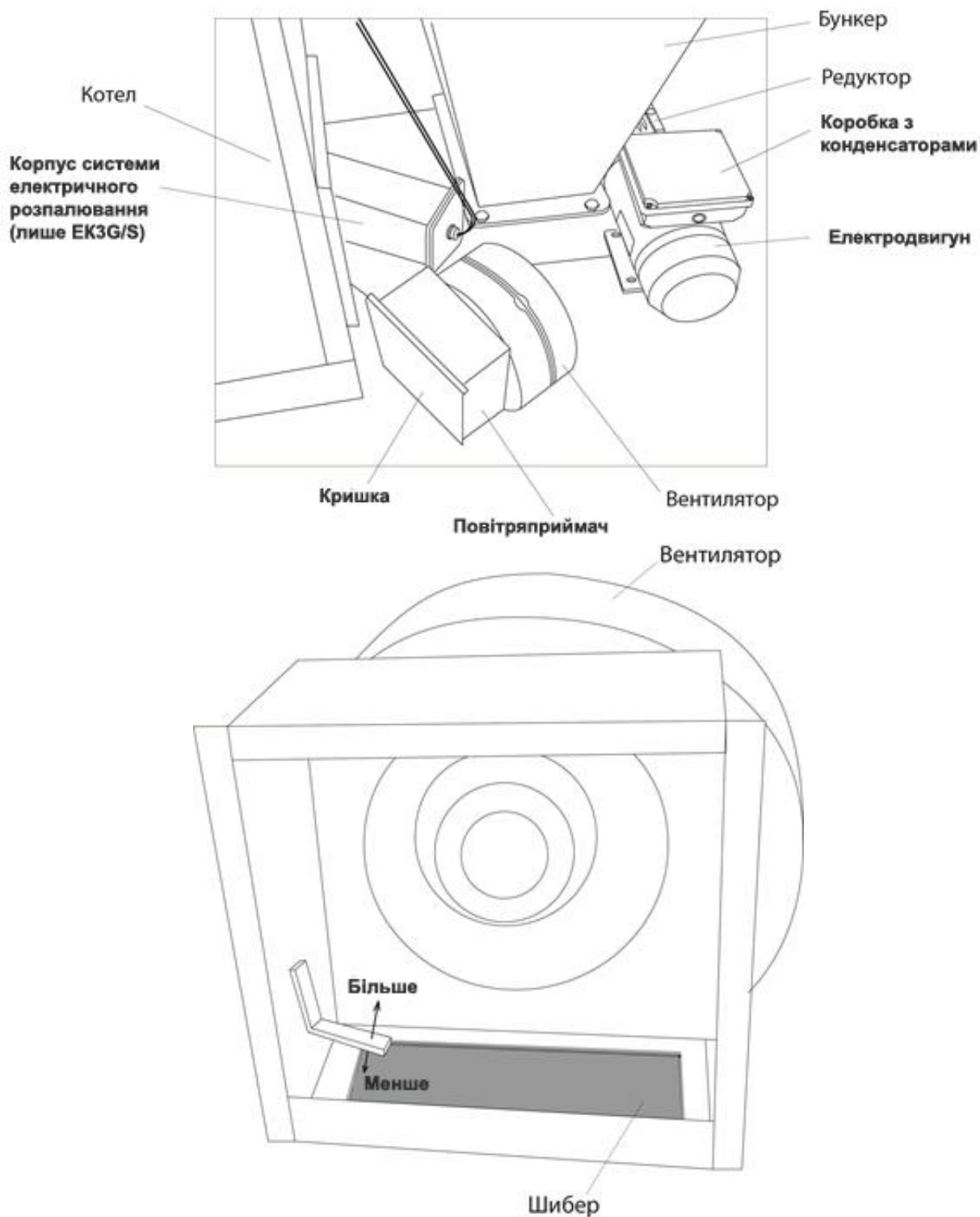
Малюнок 3 - Регулювання шиберної заслінки.
