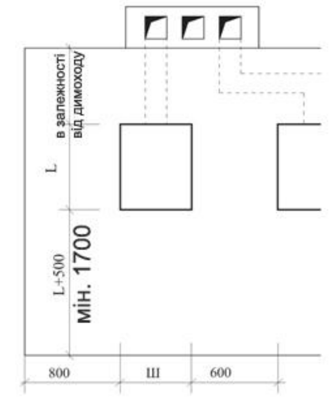
Малюнок 12 – Планування котельні.
