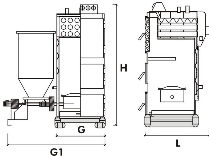
Малюнок 13 - Котел K3G/S 30-100
