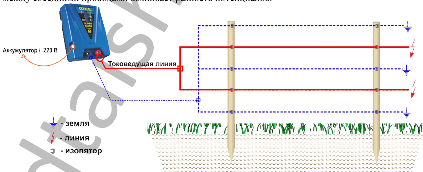
Рис. 5. Электроизгородь для районов с высоким удельным электросопротивлением верхнего слоя почвы (пески, сухие почвы, снег)
