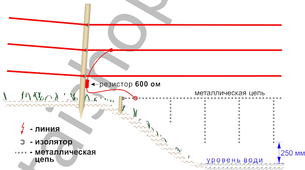
Рис. 10. Пересечение электроизгороди с водотоком
