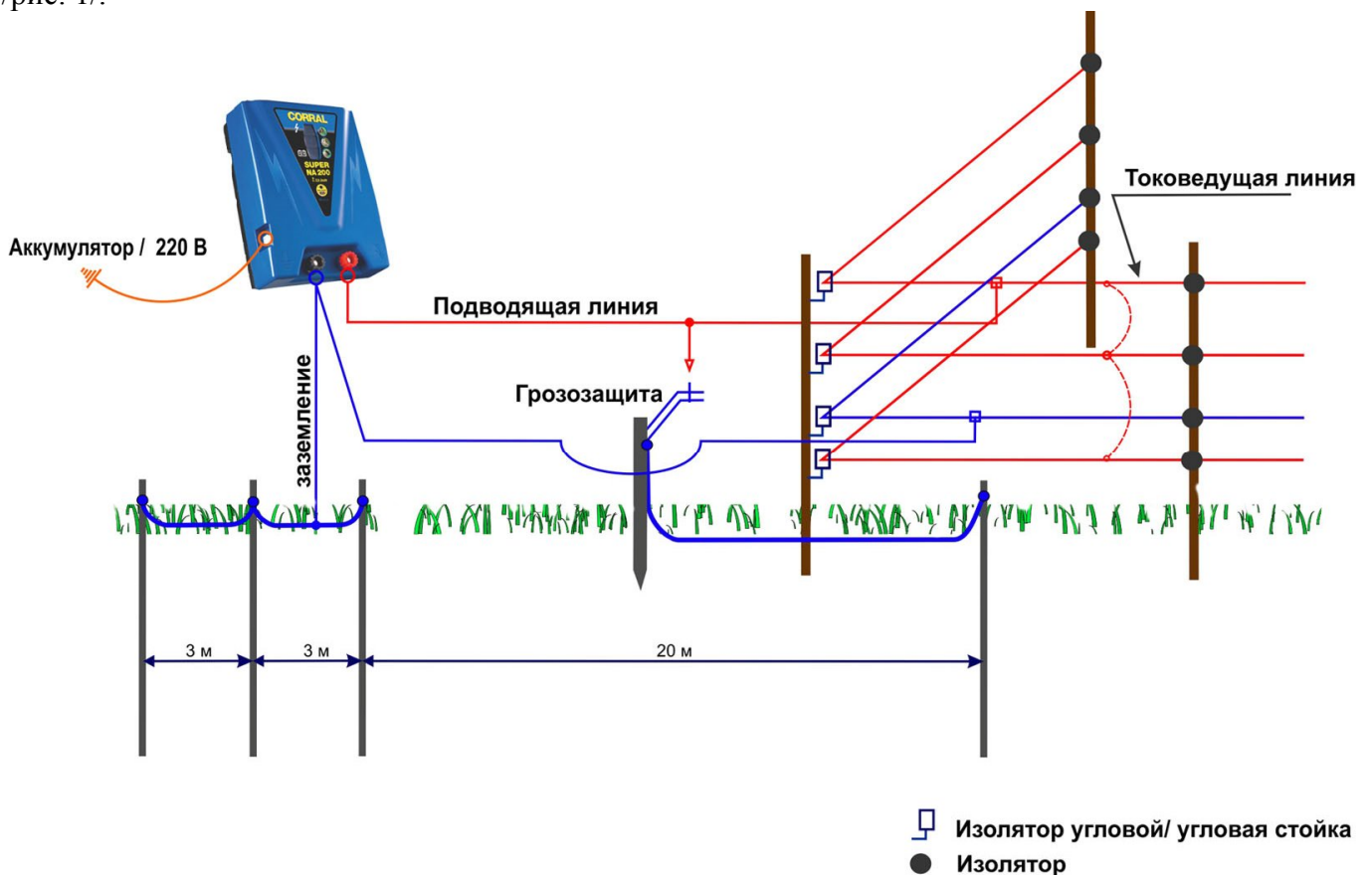
Рис. 1. Конструктивные элементы электрической изгороди
