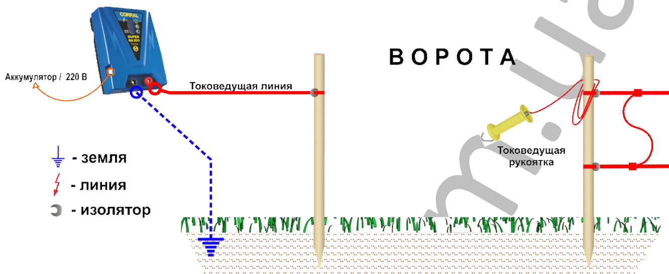
Рис. 11. Расположение токосъемной (воротной) рукоятки при устройстве ворот
