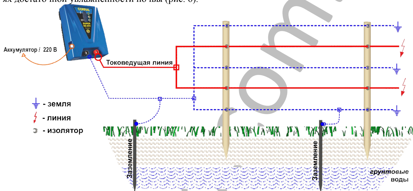
Рис. 6. Электроизгородь для районов с увлажненными почвами (более 700 мм осадков в год)
