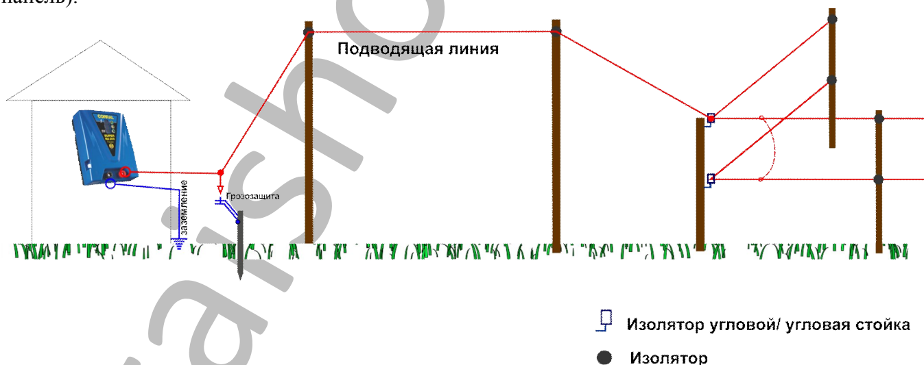
Рис. 2. Воздушная подводящая линия
