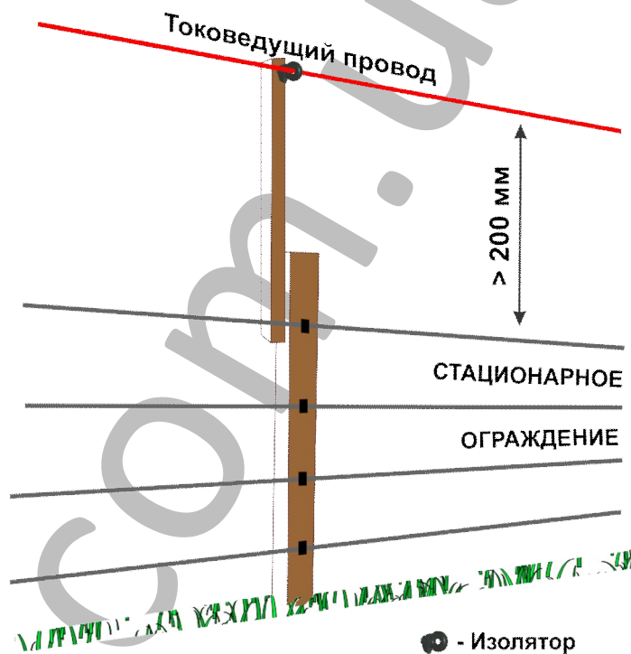
Рис. 3. Подводящая линия (вариант)
