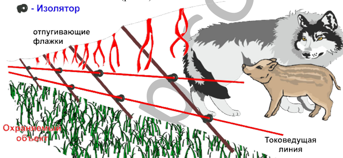
Рис. 8. Электропленочная изгородь для защиты сельхозполей от кабанов/диких животных.
