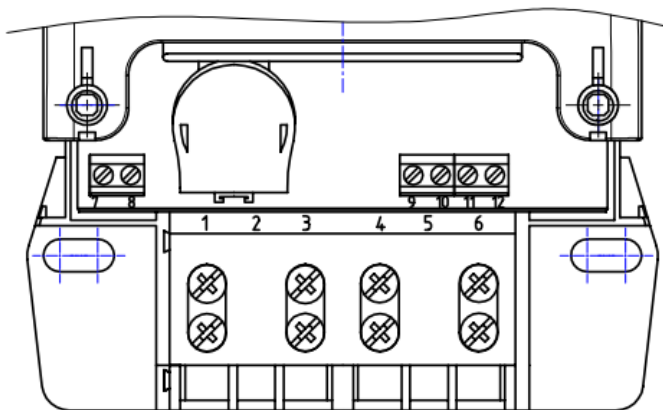
Рисунок 2.4 – Нумерация контактов счетчика CE102M S7
