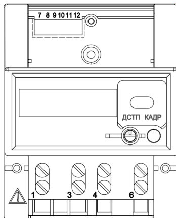
Рисунок 2.5 – Нумерация контактов счетчика CE102M R5
