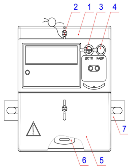
Рисунок 2.3 Внешний вид счетчика CE 102M R5.1
