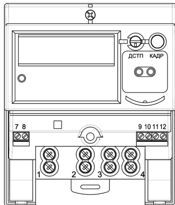
Рисунок 2.6 – Нумерация контактов счетчика CE102M R5.1
