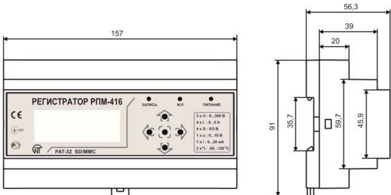
Рисунок 3.1 – Внешний вид и габаритные размеры регистратора
