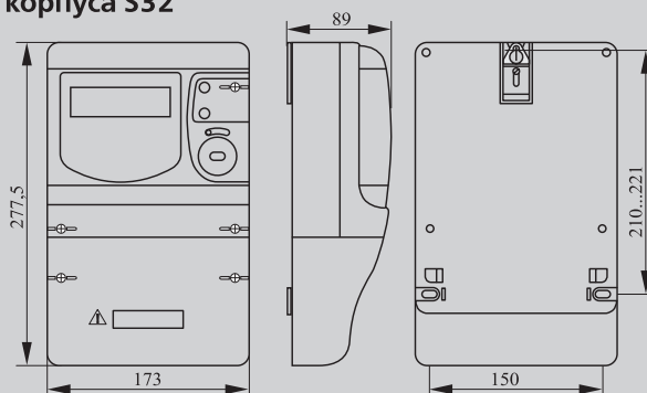
Тип корпуса S32
