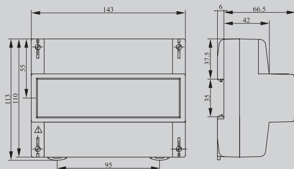
Тип корпуса R5.1.
