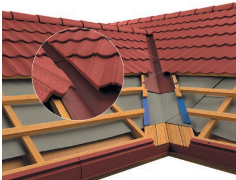
РИС. 26 Монтаж ендовы
