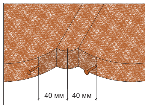
Узел 1
