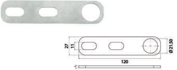
Bağlantı Sacı CNG 01 Connection Steel CNG 01
