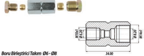
Boru Birleştirici Takım Ø6 - Ø8 Pipe Coupling Set Ø6 - Ø8
