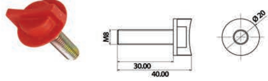
M8 x 30 mm Kaplamalı Civata M8 x 30 mm Covered Screw
