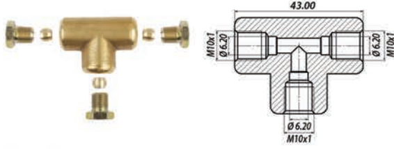
T Takım Ø6 x Ø6 x Ø6 T Set Ø6 x Ø6 x Ø6
