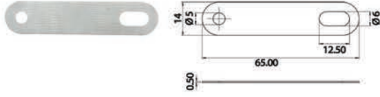
Bakır Boru Kroşe 65,00 x 14,00 x 0,50 mm Copper Pipe Clamp 65,00 x 14,00 x 0,50 mm
