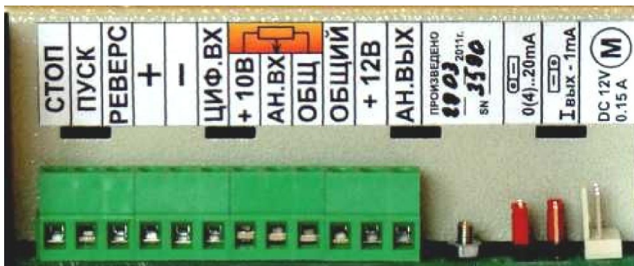
Рисунок 7 – Клеммы внешнего управления.
