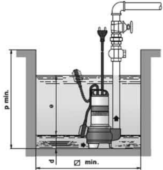
Типова установка однофазного насоса
