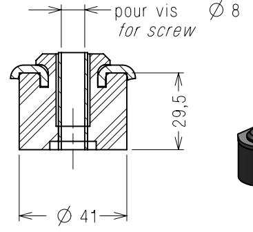
Detail suspension Echelle : 1/2 Scale : 1/2
