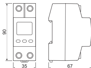
Габаритні розміри
