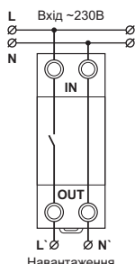
Схема підключення
