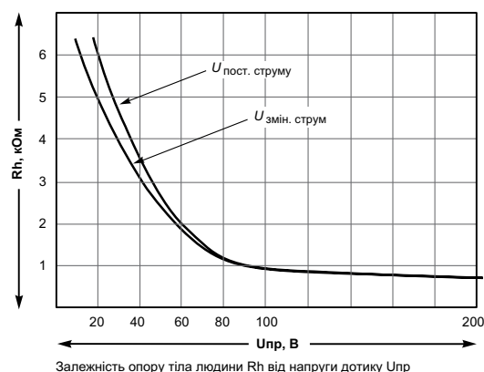
Залежність опору тіла людини R_h від напруги дотику U_{пр}
