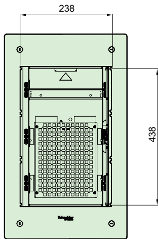
13 модулів
