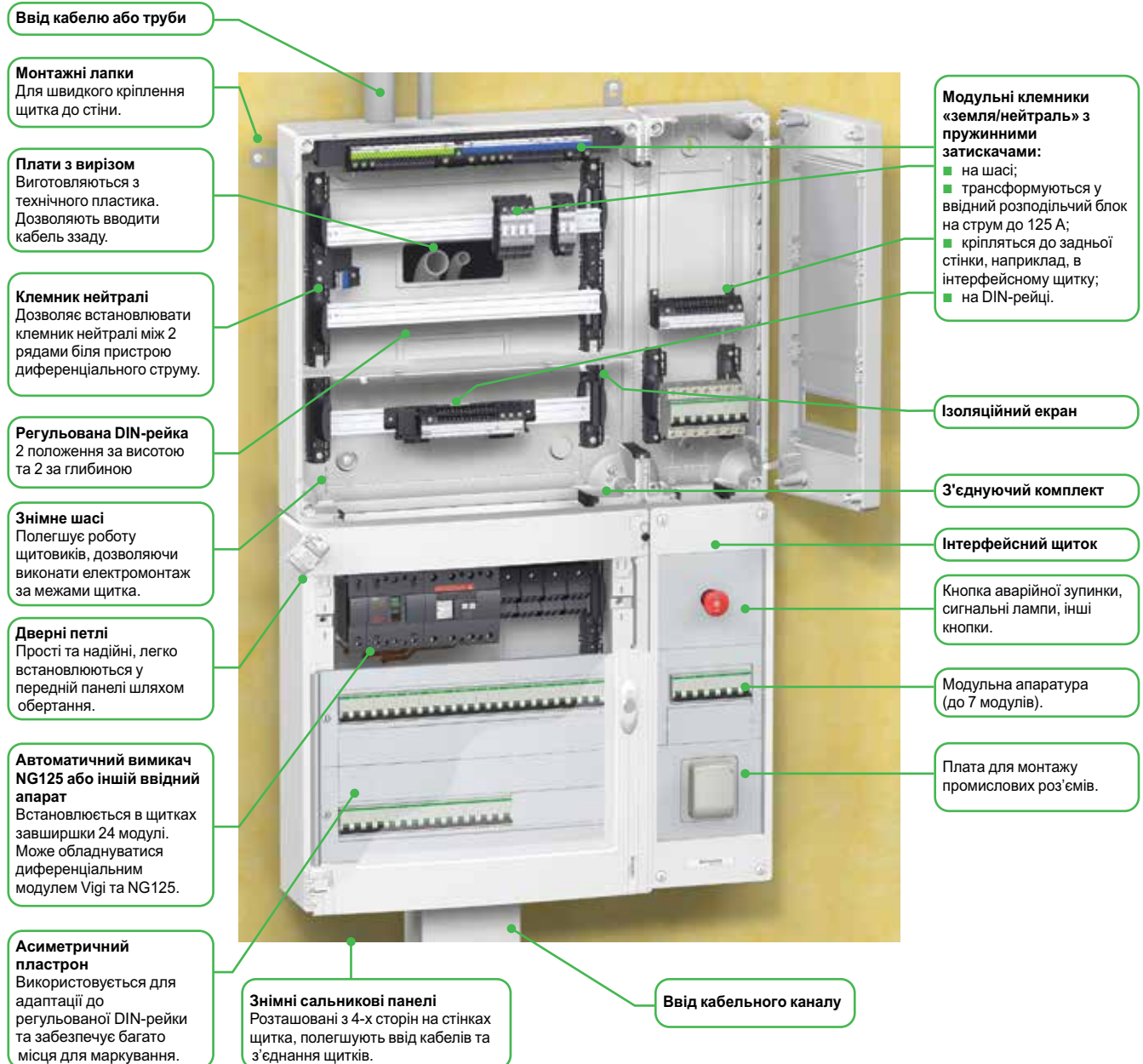
Інтерфейсний щиток
