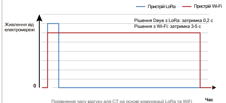
Діаграма часу відгуку функції нульового експорту
