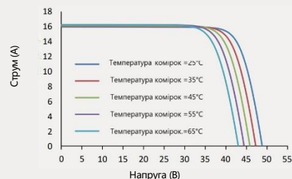
Струм-напруга (615 Вт)
