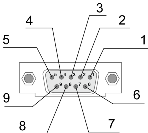
Рис. 2.5.1 Интерфейсный разъём
