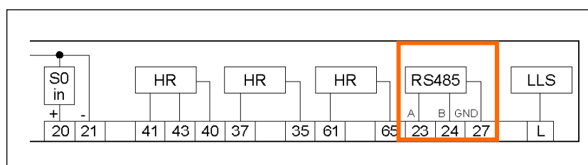
Рисунок 19: Диаграмма связей - RS485
