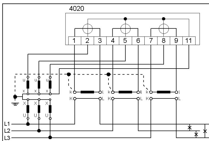
Рисунок 8: Счетчик трансформаторного включения; тип записи измерений М1 (4020)
