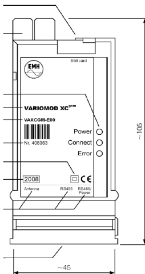
Рисунок 28: Элементы, изображенные на корпусе
