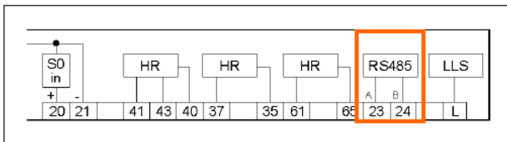
Рисунок 19: Диаграмма связей - RS485
