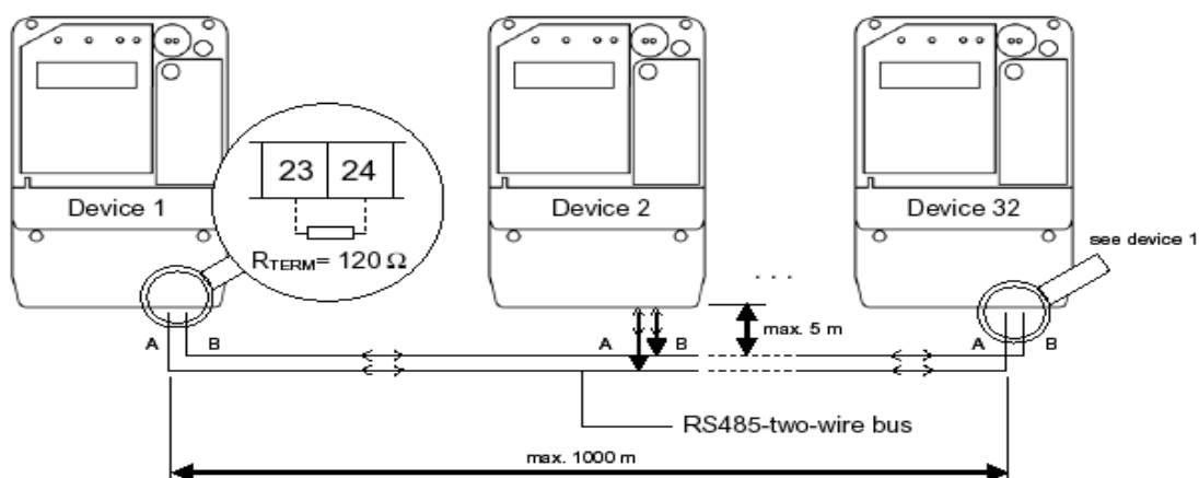
Рисунок 21: RS-485-двухпроводная система шины
