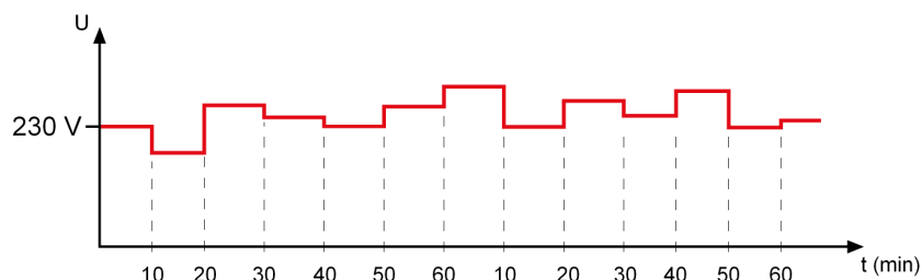
Рисунок 38: Диаграмма дополнительного профиля нагрузки
