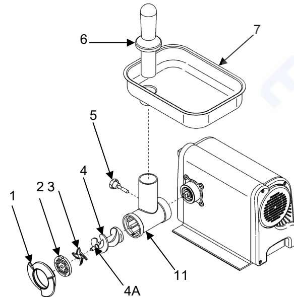
Мал. 10а - Демонтаж компонентів ТЗ
