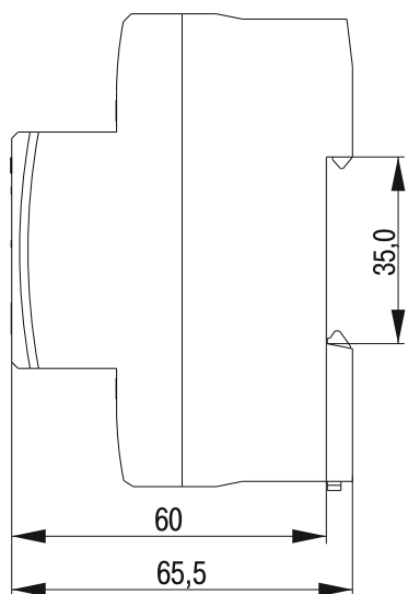
Рисунок 2 - Габаритні та настановні розміри реле
