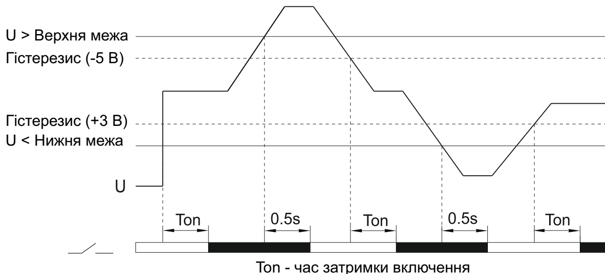
Рисунок 4 - Діаграма напруги реле
