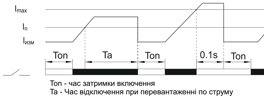
Рисунок 5 - Діаграма струму реле
