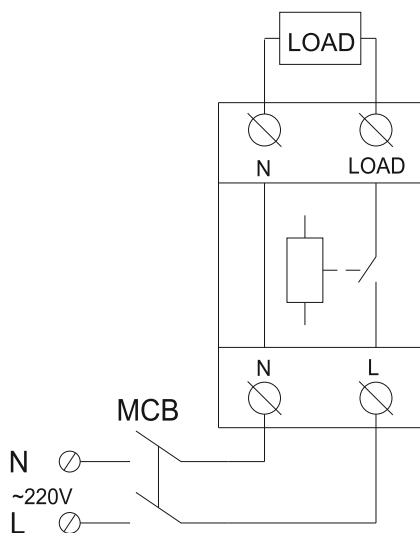
Рисунок 3 - Умовна схема підключення реле
