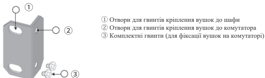
Рисунок 2-2. Схема зовнішнього вигляду монтажних вушок
