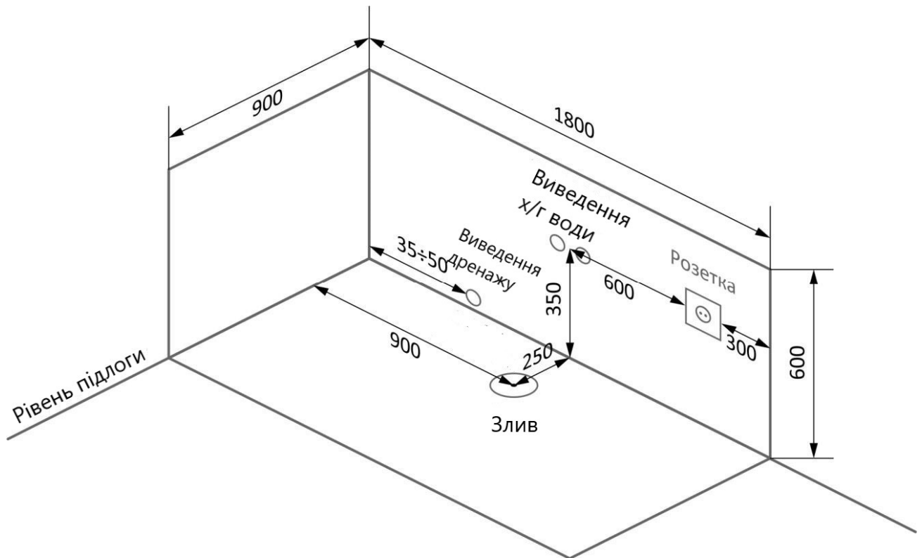
Схема 3. Підведення комунікацій, мм
