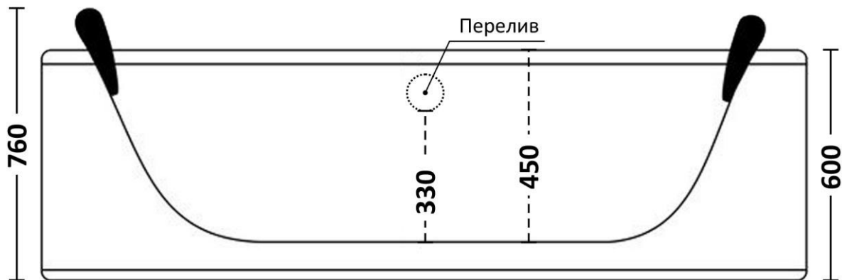
Схема 2. Габаритні розміри Iris TLP-658, мм
