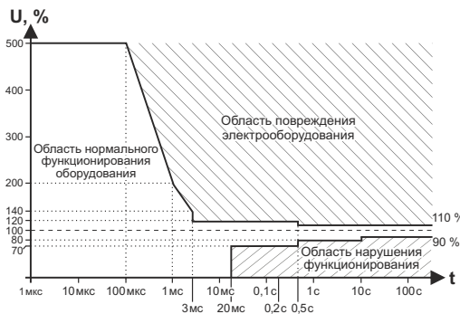
Рис. 1. Кривая работы датчика электрооборудования ITIC (CBEMA), ( http://www.home.agilent.com/upload/cmcc_upload/All/1.pdf?&cc=UA&lc=eng ).
