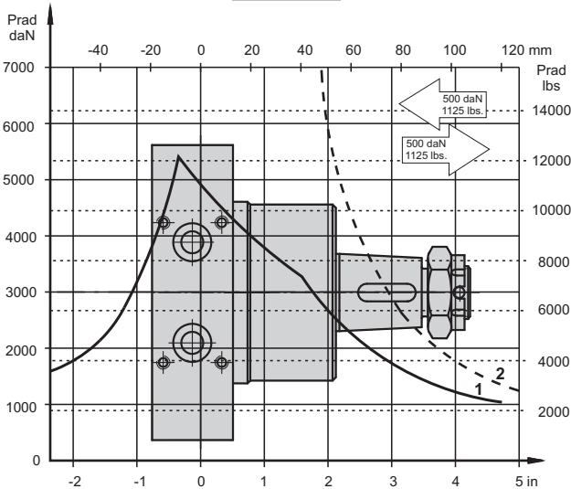
HWV...
