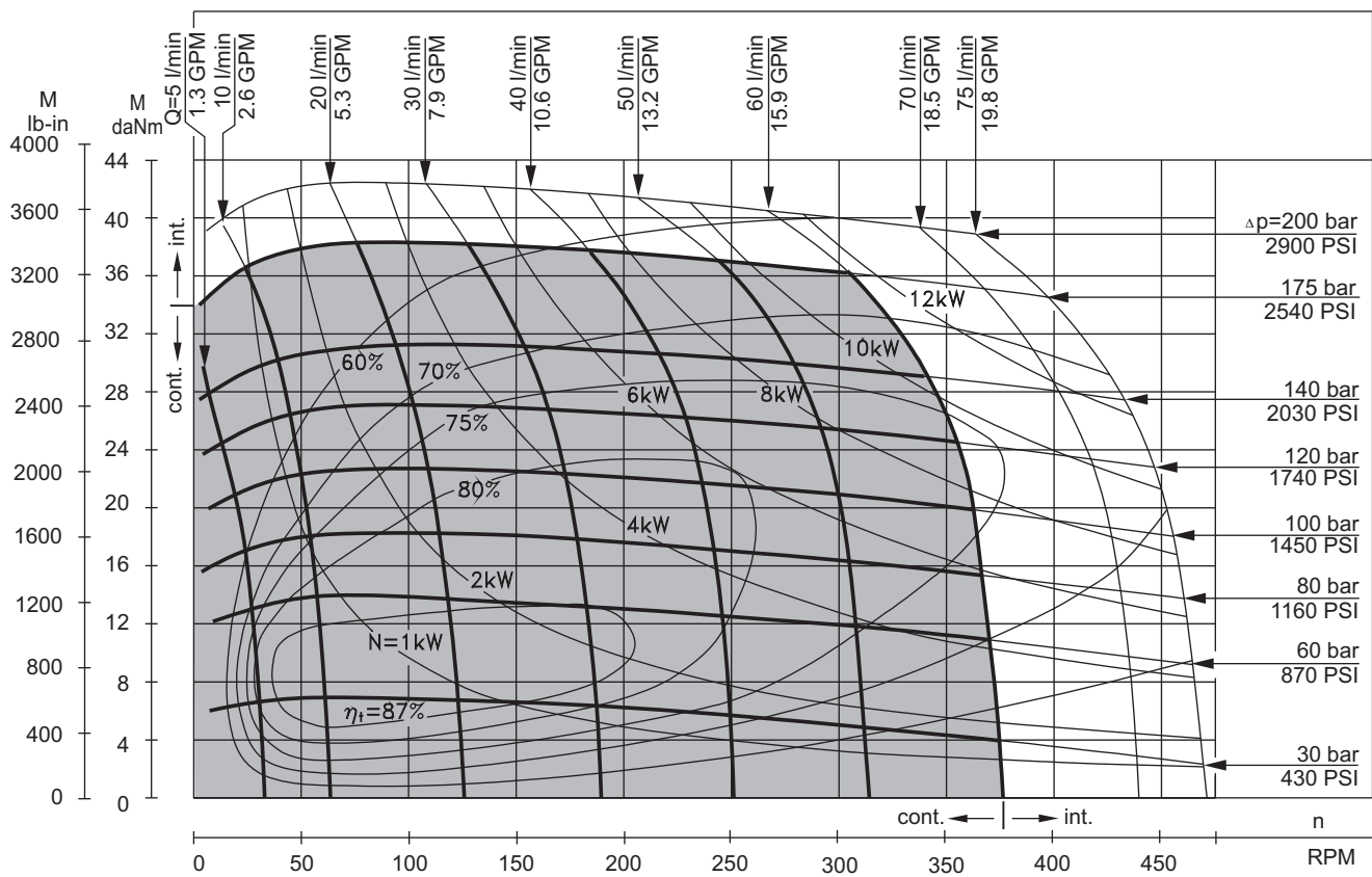
RW 160
