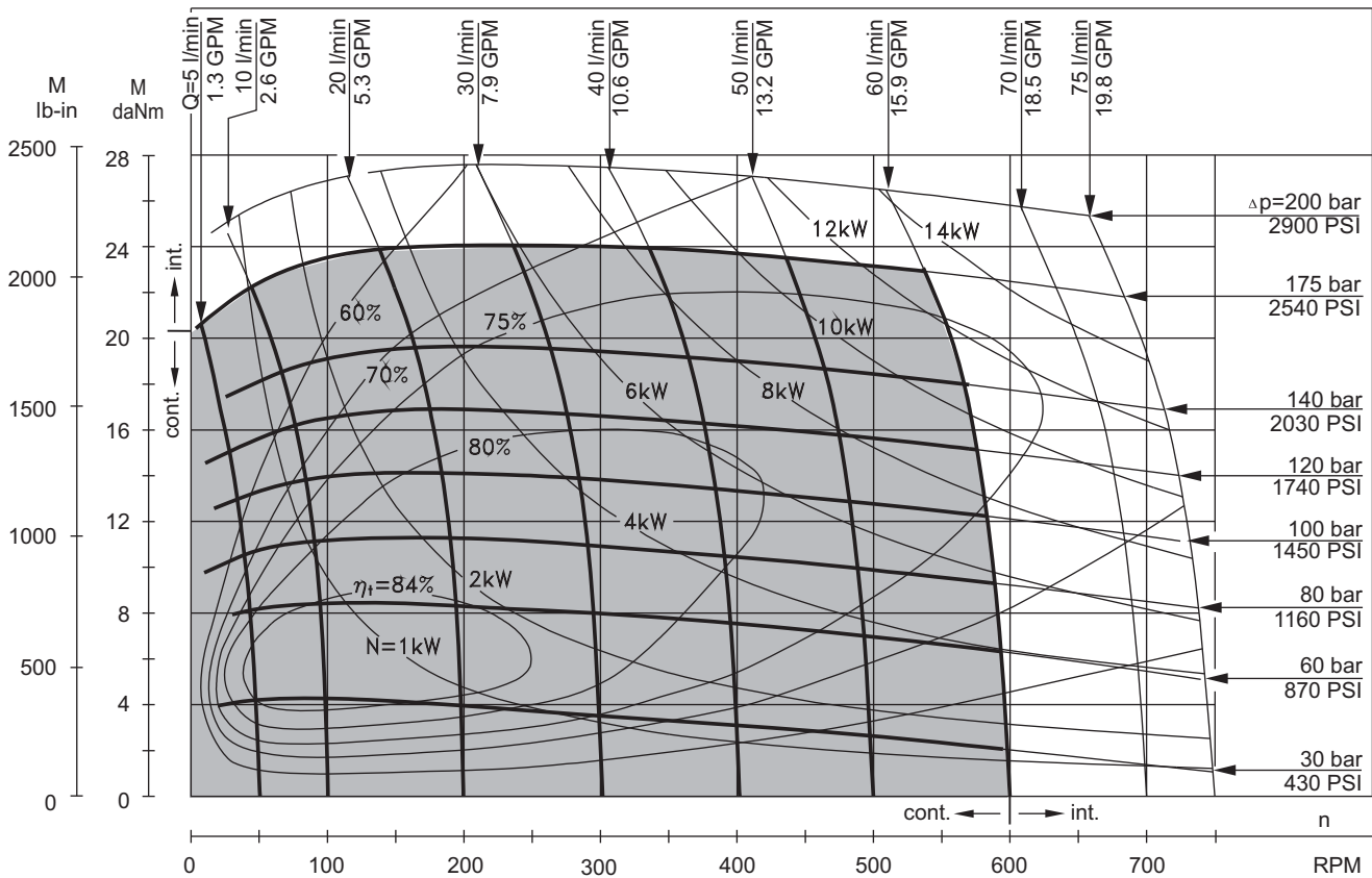
RW 100
