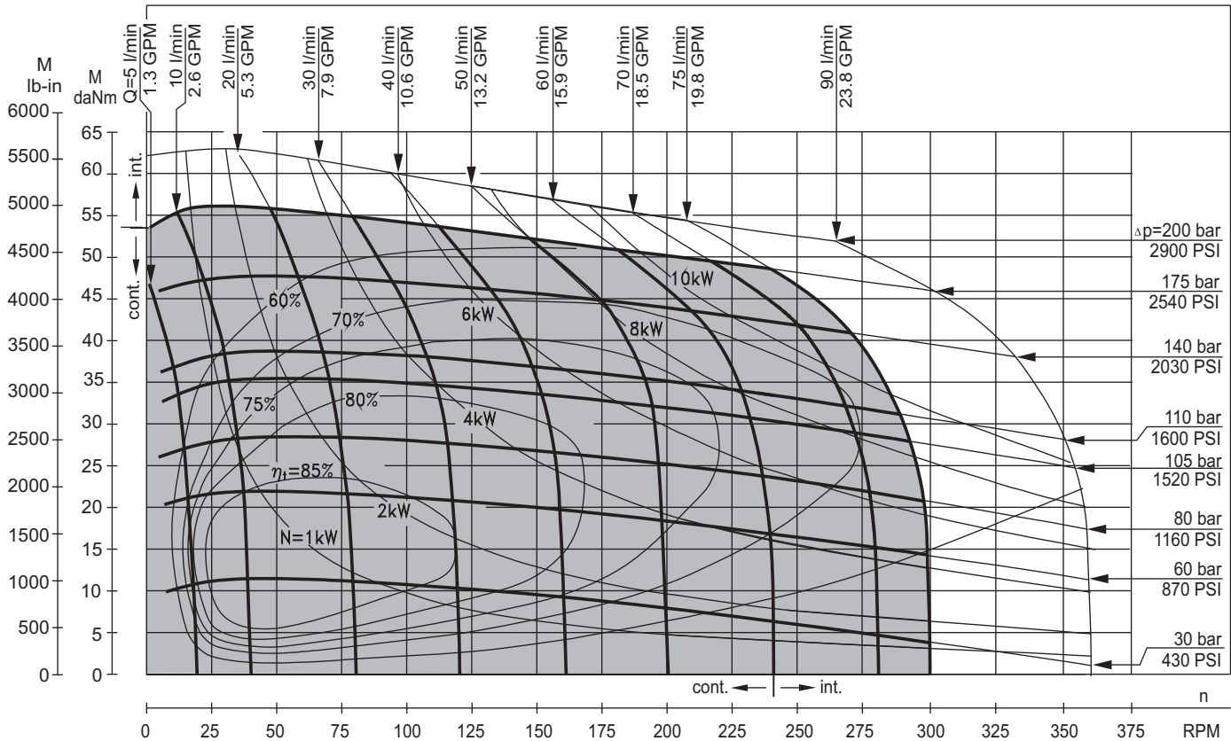
RW 315
