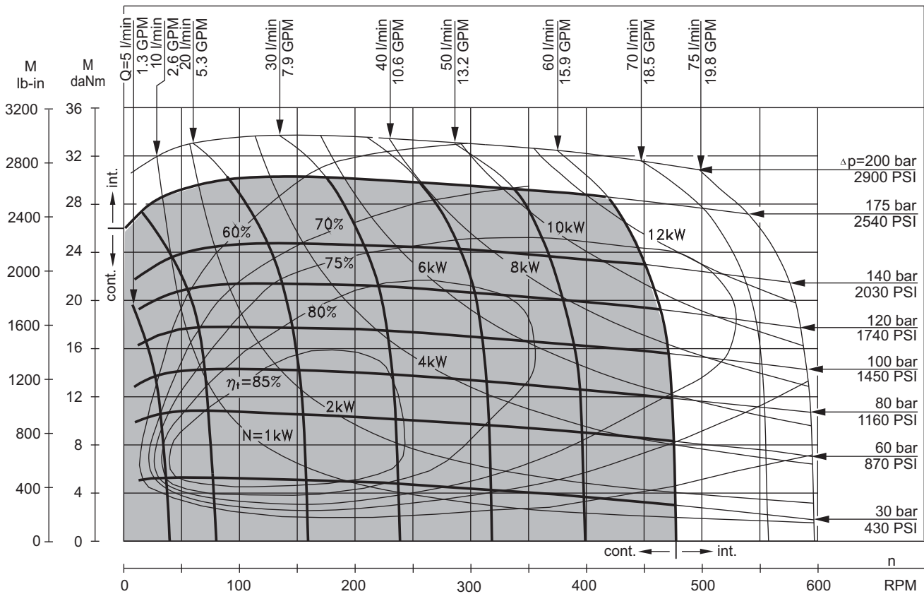
RW 125
