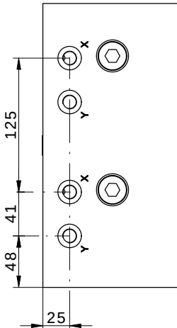
C019 RELIEF VALVE
