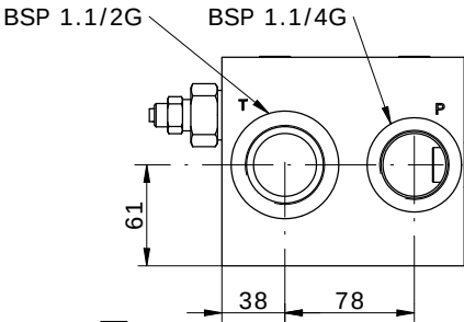
C019 RELIEF VALVE
