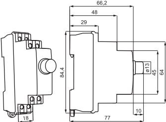
MBF (з фіксацією)
