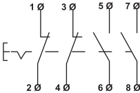
Модульна кнопка з фіксацією MBF
