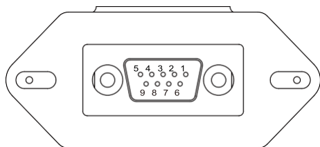
DB9 (RS232)
