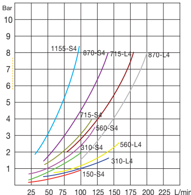
Diagramma perdite di carico/Pressure drop
