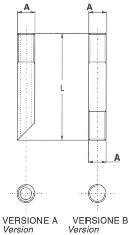
Tubo di scarico per filtri FTT Clearance tube for FTT filter
