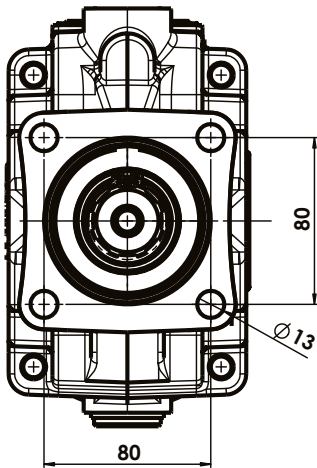
ISO 3019-1 SAE C - 4fori / holes
