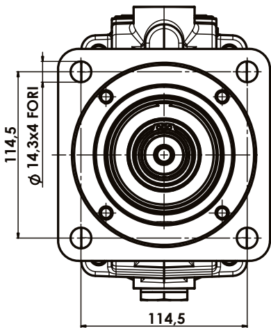
ISO 3019-1 SAE C - 4fori / holes
