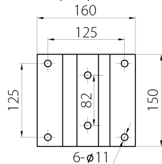
Розміри кронштейна
