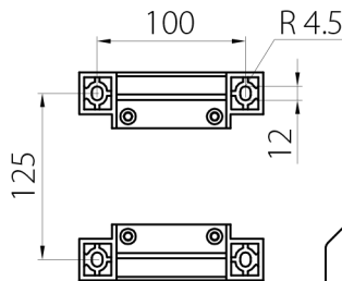
Розміри кронштейна
