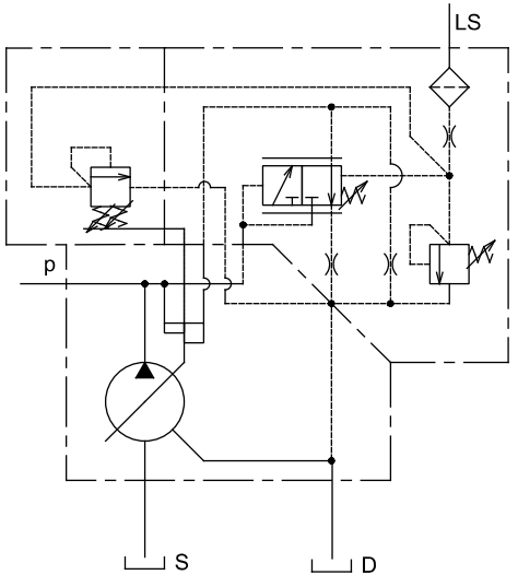
Schema idraulico pompa con regolatore PW Pump with PW control hydraulic scheme
