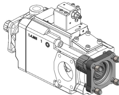
11465000137 Applicazione PPV tandem 130-150 / Pompa ISO 7653 (coppia trasmissibile 800 Nm) PPV tandem 130-150 size / ISO 7653 pump adaptor (Max. allowed torque 800 Nm)
