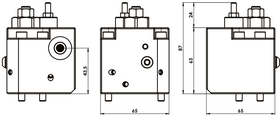
Ingombro / Dimensions
