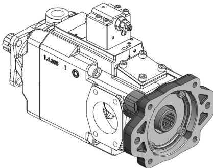
11465010420 Applicazione PPV tandem 130-150 / Pompa SAE C Z14 (coppia trasmissibile 640 Nm) PPV tandem 130-150 size / SAE C Z14 pump adaptor (Max. allowed torque 640 Nm)
