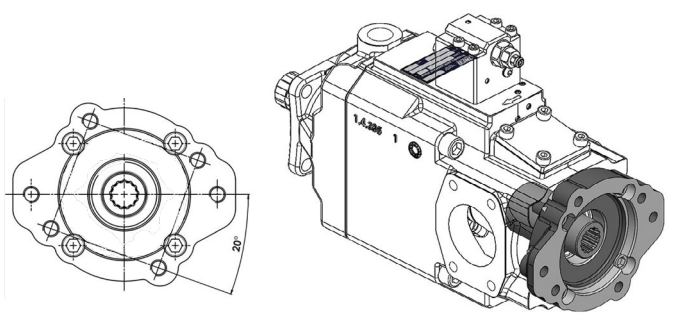
11465010322 Applicazione PPV tandem 130-150 / Pompa SAE BB Z15 (coppia trasmissibile 400 Nm) PPV tandem 130-150 size / SAE BB Z15 pump adaptor (Max. allowed torque 400 Nm)
