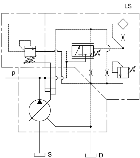
Schema idraulico pompa con regolatore PW Pump with PW control hydraulik scheme
