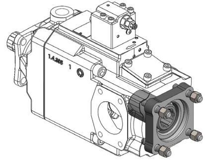
11465000137 Applicazione PPV tandem 130-150 / Pompa ISO 7653 (coppia trasmissibile 800 Nm) PPV tandem 130-150 size / ISO 7653 pump adaptor (Max. allowed torque 800 Nm)
