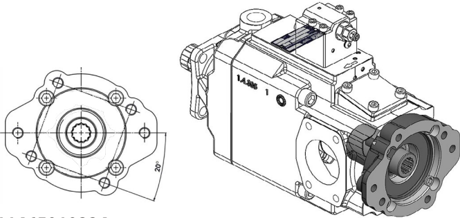
11465010224 Applicazione PPV tandem 130-150 / Pompa SAE B Z13 (coppia trasmissibile 210 Nm) PPV tandem 130-150 size / SAE B Z13 pump adaptor (max. allowed torque 210 Nm)
