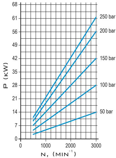
MGP2.5K45
