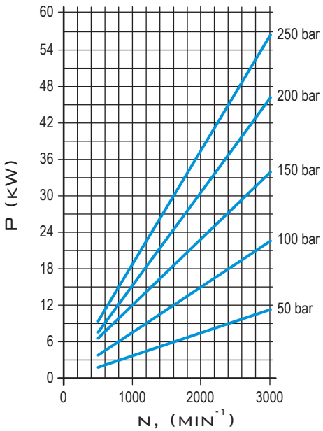
MGP2.5K36
