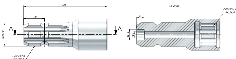
ARA UZATMA| ISO - ASAE ADAPTER
