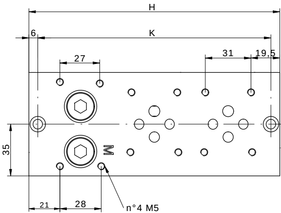
INTERFACCIA AUSILIARE SU ELEMENTI AGGIUNTIVI (USARE OR2106) INTERFACE FOR ADDITIONAL AUXILIARY ELEMENTS (USE OR2106)
