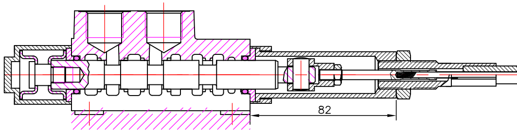
P80 A1G V1(l= . . .)+ 3047 Spool valve / Zawór suwakowy Kabel / Przewód Control body / Sterowanie obudową
