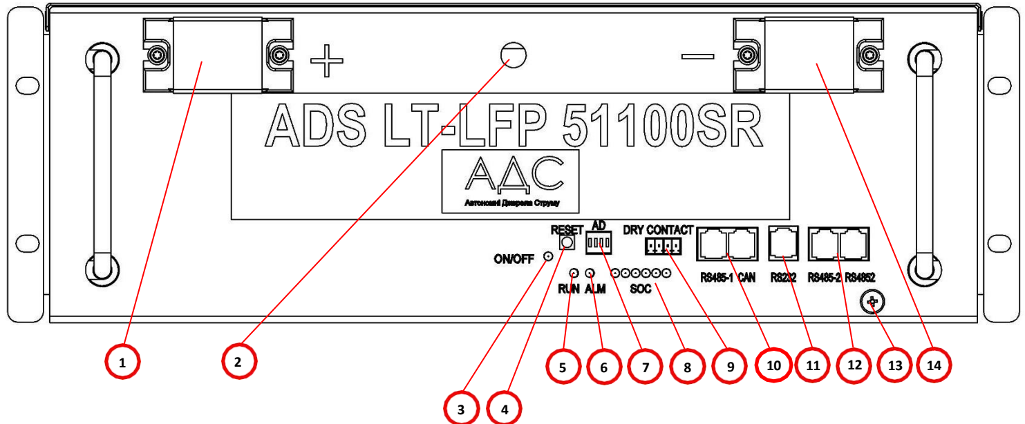
Рис.2-3 Зображення панелі управління
