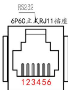
Таблиця 2-6 Визначення інтерфейсу RS232
