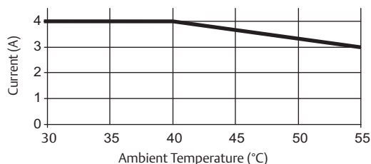
Макс. ток в зависимости от темп. окружающей среды
