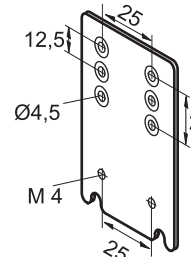
Удлинительная скоба
