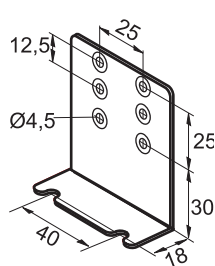
Монтажная скоба угловая
