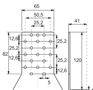
Универсальная скоба
